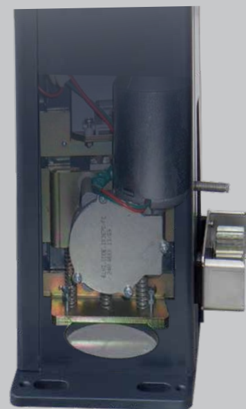
Motorisation invisible intégrée dans le pilier de guidage
